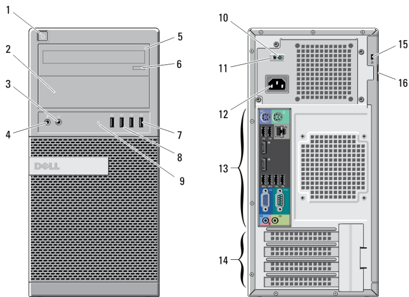
Slika 1. Prikaz sa prednje i zadnje strane za Mini-Tower kućište
